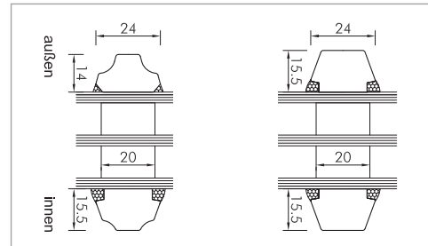
Einsetzfräsung im Rahmen
