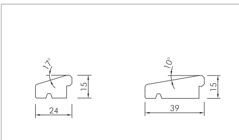
Eingenuteter Wetterschenkel
