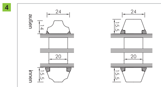
Sprossen – 2 Falzarten:
