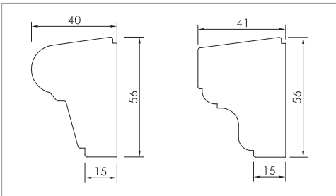
Kämpferprofile **
