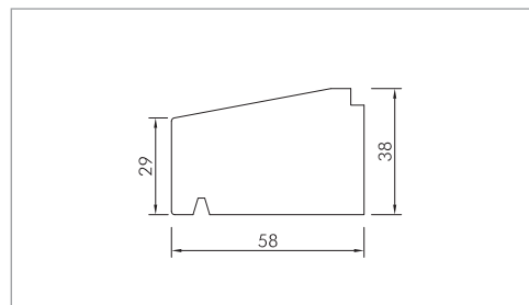
Sohlbankprofil **
