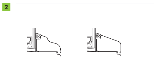
Glasleiste – 2 Falzarten:
