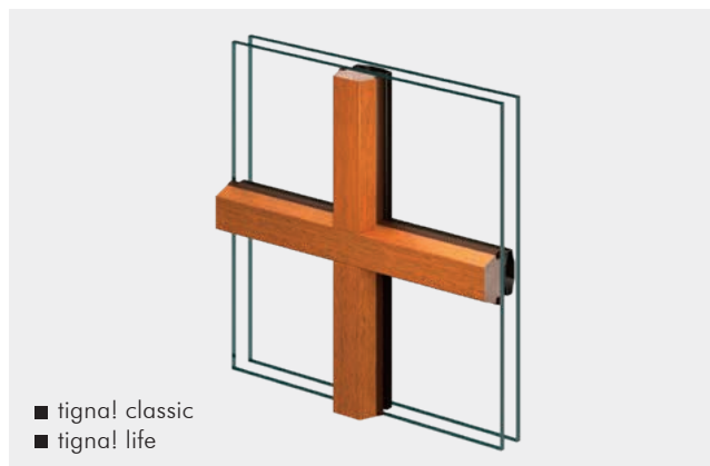
Einseitig aufgesetzte Trapezfalzsprosse/Alu-Sprosse im Scheibenzwischenraum (28 mm)
