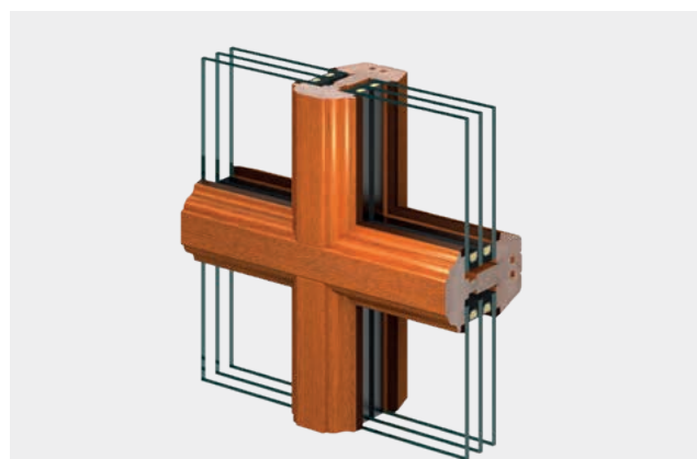
Glasteilende Zierfalzsprosse (48 mm), Trapezfalzsprosse innen
